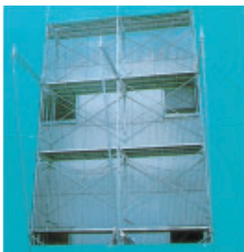
斜材を持ち上げピンをセットし、カブラを仮止め
